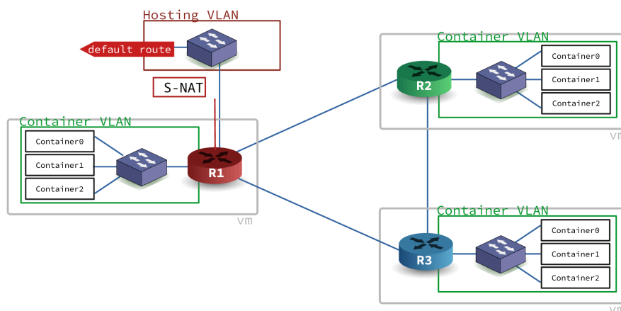
Topologie logique en triangle
